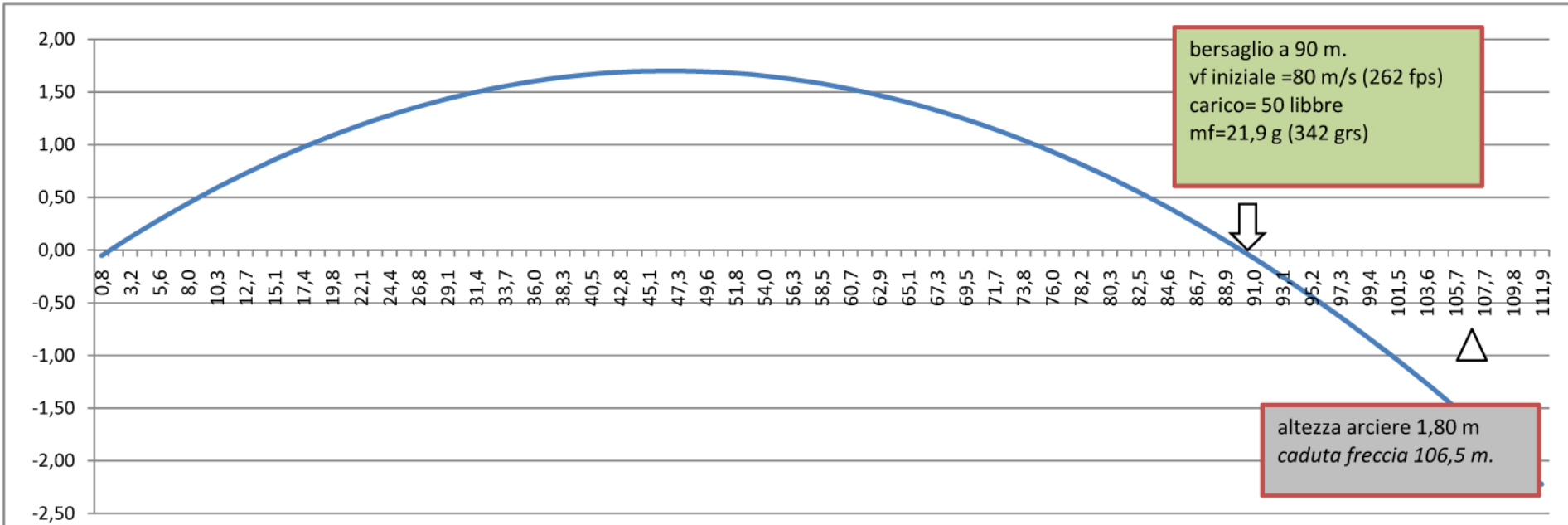
Grafico 1 (errore di brandeggio)
